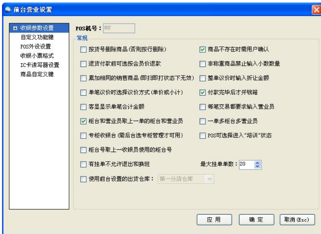
图 收银参数设置-常规
