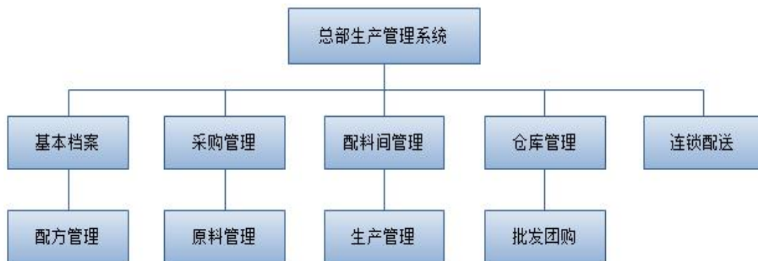
图 生产管理系统功能结构图
