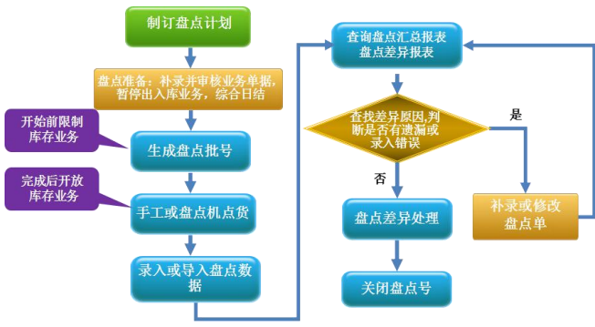
图 盘点流程
